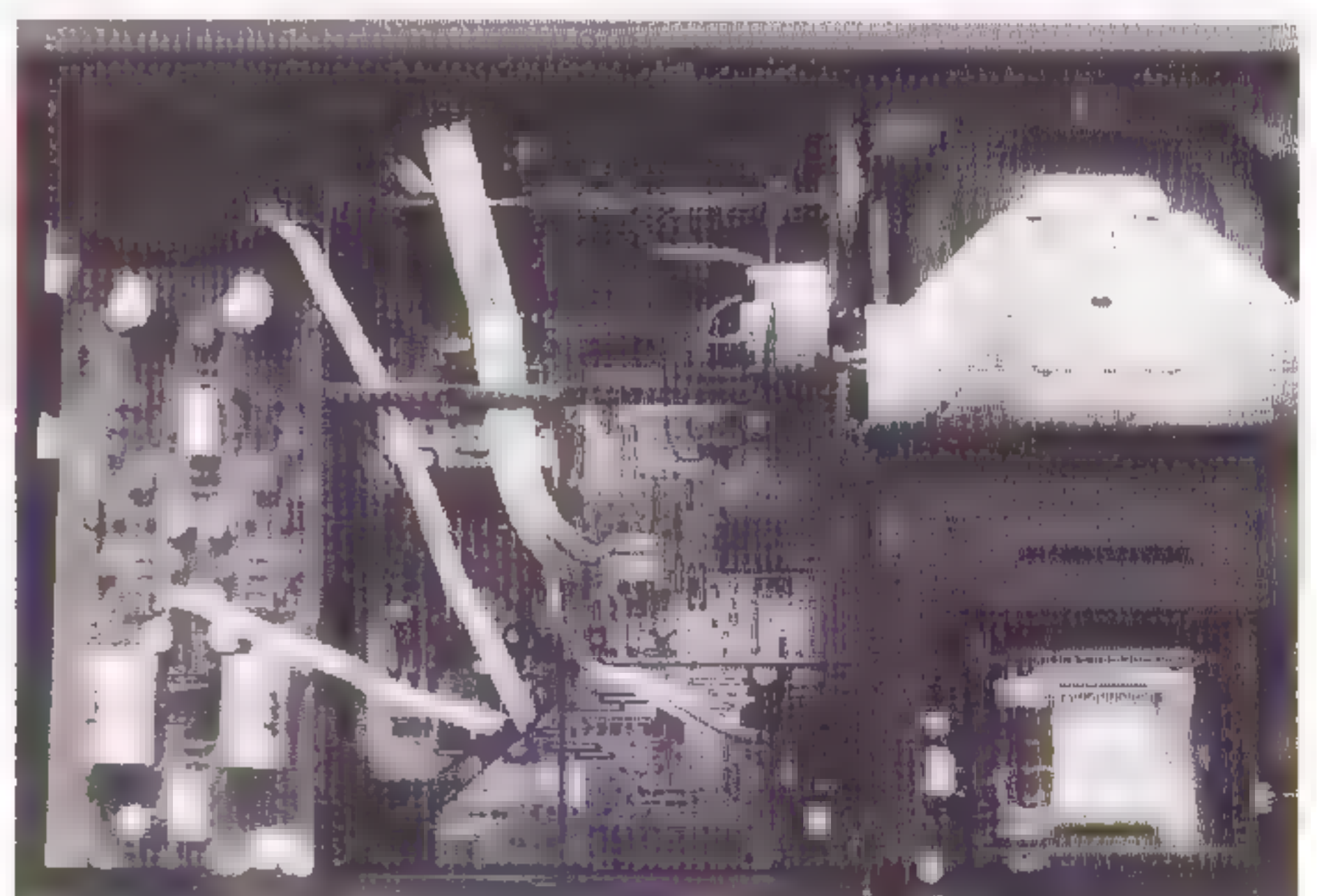
Links is de binnenkant van de standaard Marantz CD-40 te zien en rechts het gemodificeerde exemplaar. Duidelijk zichtbaar is de nieuwe printplaat met de grote MKP uitgangscondensatoren.
